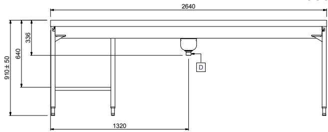
Alzado
